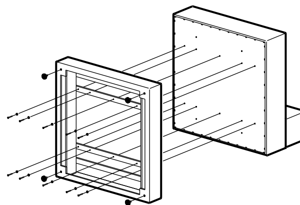
BOX Leg 組立
