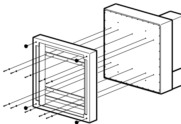
BOX Leg 組立
