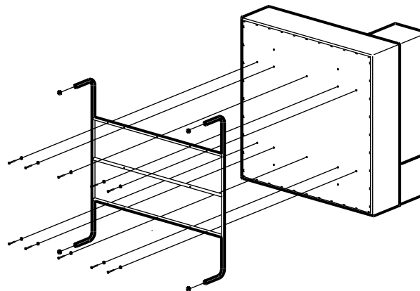
BEND Leg 組立
